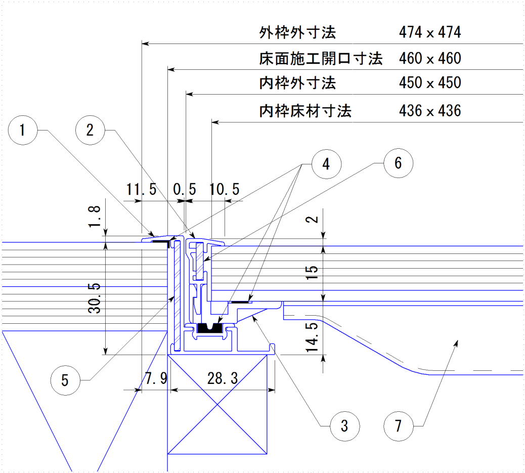
断面詳細
