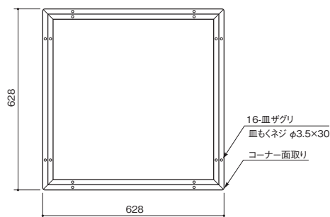
■仕様図
