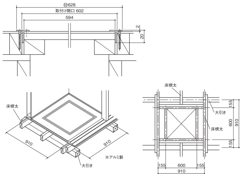
■取付図
