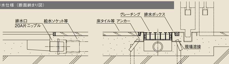
端部排水仕様 (断面納まり図)
