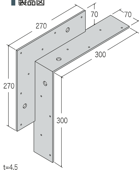
■ 製品図
