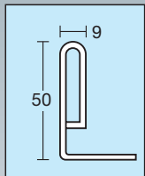
●棚板断面図
