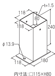
内寸法: □115×H80
