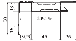
※( )内寸法はFV-NEC1226KF-L09
