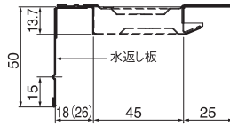
※( )内寸法はFV-NEC0826KF-L09
