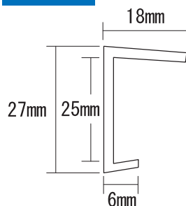
詳細図
