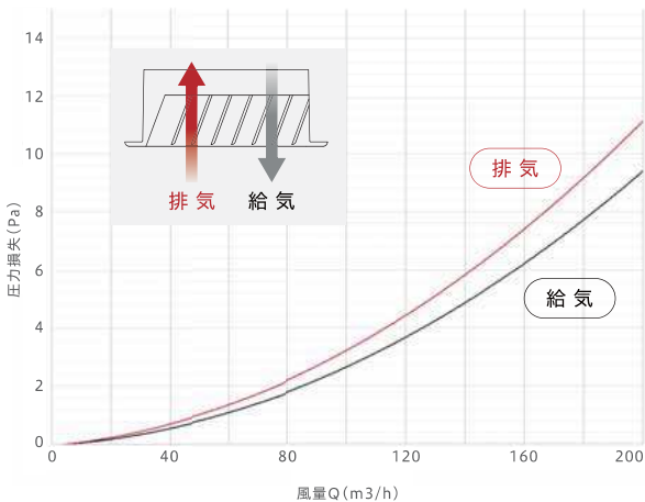
P-Q特性図
