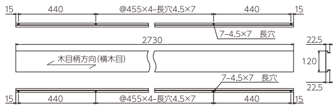
PW-TM12025-L27の寸法図
