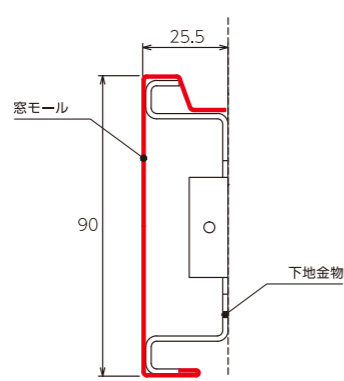
PW-MM9025-L27の納まり図
