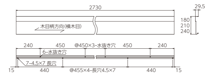
PW-YM18030-L27 PW-YM21030-L27 PW-YM24030-L27の寸法図
