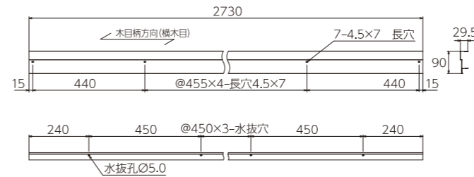
PW-DM9030-L27の寸法図
