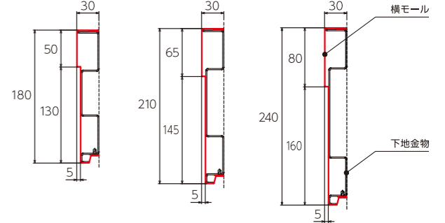
PW-YM18030-L27 PW-YM21030-L27 PW-YM24030-L27の納まり図
