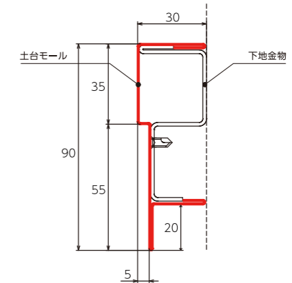
PW-DM9030-L27の納まり図
