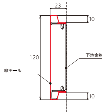
PW-TM12025-L27の納まり図
