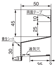
WMF-N50(出幅50mm)
