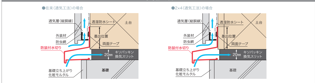
参考納まり図
