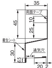
WMF-N35(出幅35mm)
