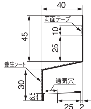
WMF-N40(出幅40mm)
