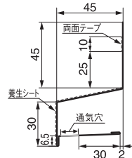
WMF-N45(出幅45mm)
