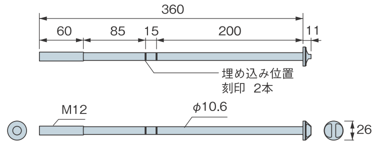
■寸法図 (M12)
