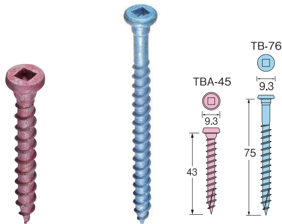
TBA-45 柱側 (使用本数2本)
