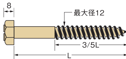
■寸法図
