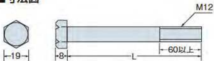
■寸法図
