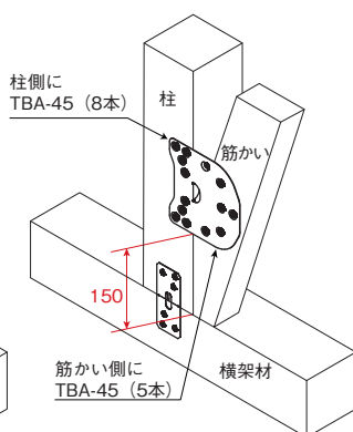
45mm×90mmの筋かい接合
