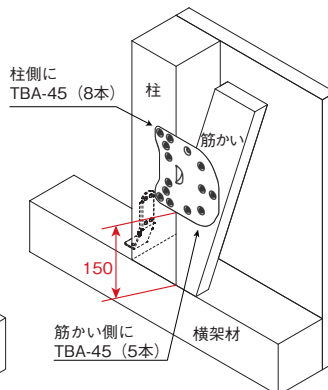
30mm×90mmの筋かい接合※ (リフォーム時)
