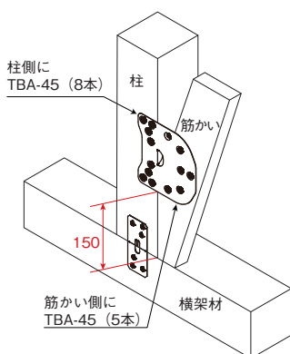
30mm×90mmの筋かい接合※
