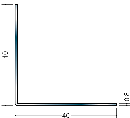
20034 ステンアングル 0.8×40×40 3m/ヘアライン
