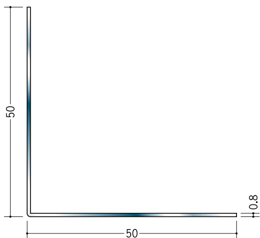
20047 ステンアングル 0.8×50×50 3m/ヘアライン
