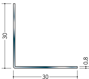
20033 ステンアングル 0.8×30×30 3m/ヘアライン
