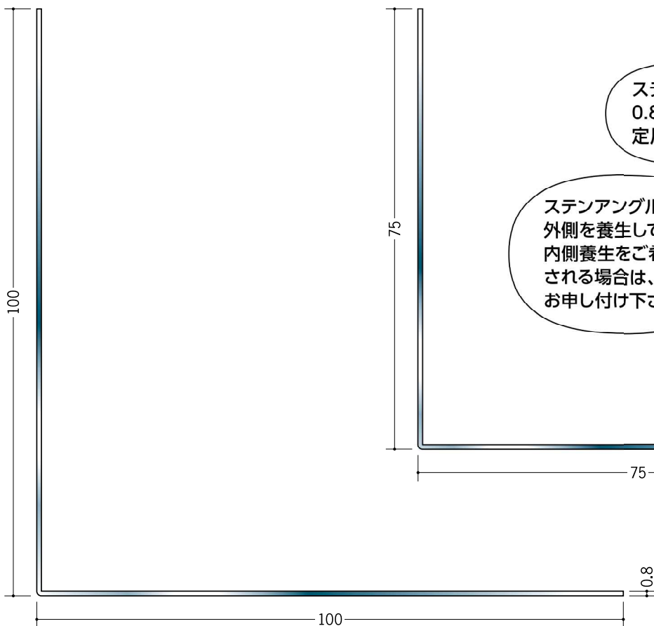
63142 ステンアングル 0.8×100×100 3m/ヘアライン
