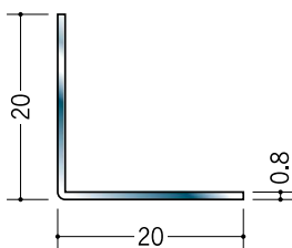
20031 ステンアングル 0.8×20×20 3m/ヘアライン
