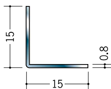
20030 ステンアングル 0.8×15×15 3m/ヘアライン
