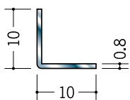
20029 ステンアングル 0.8×10×10 2m/ヘアライン
