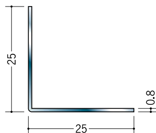
20032 ステンアングル 0.8×25×25 3m/ヘアライン
