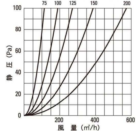
圧力損失曲線(水止め付)
