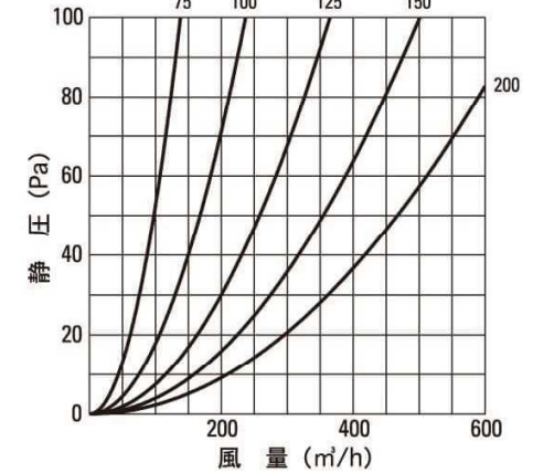
圧力損失曲線(水止め付)
