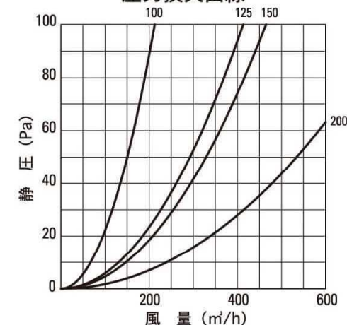
圧力損失曲線
