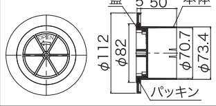
PKクーラースリーブ用 キャップφ75
