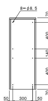
背面図
