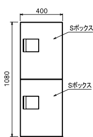
TBX-G2S(-G)ユニット
