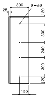
側面図
