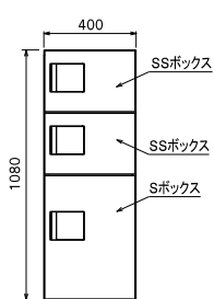
TBX-G2SS(-G)ユニット
