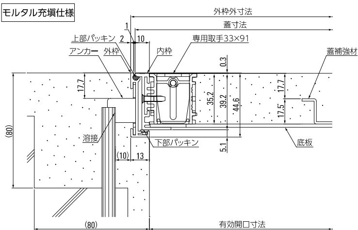
納まり図
