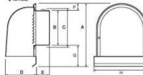
寸法図
