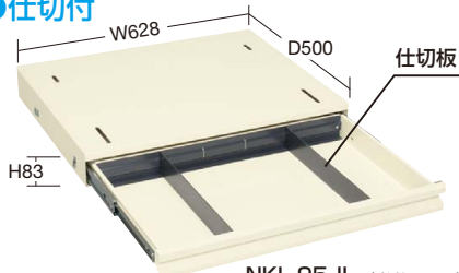
NKL-95JI (単位: mm)
