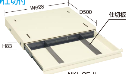
NKL-95JI (単位: mm)
