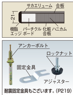
●天板断面図
