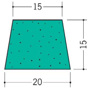
07070 EMS-30 2m / 50本入
