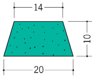
07069 EM-25 2m / 50本入
