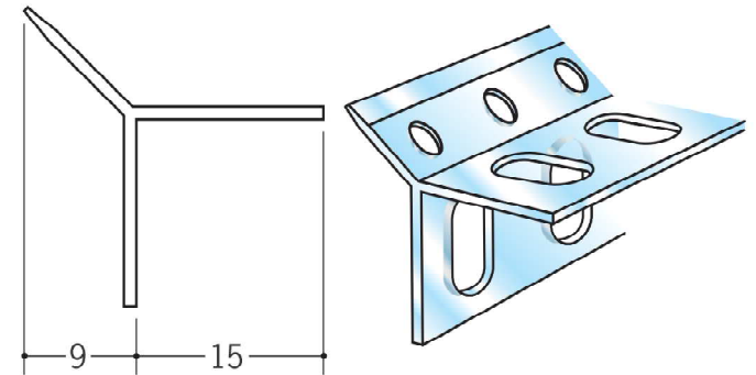
04008 かど定木D-9 1.82m/半透明/100本入
