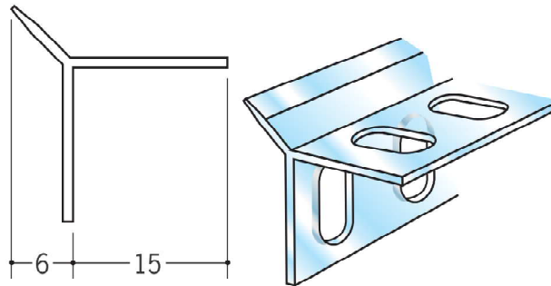
04019 かど定木D-6 1.82m/半透明/150本入
