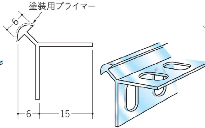
04017 かど定木A-6 プライマー付 1.82m/半透明/150本入
