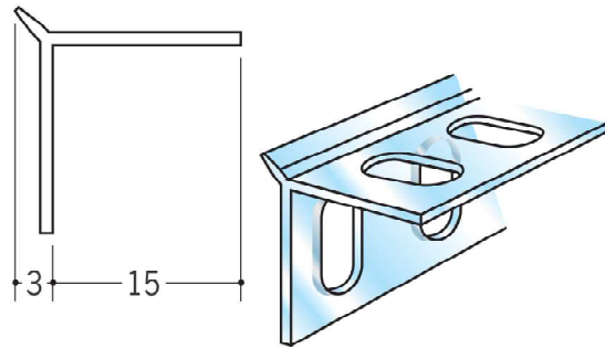
04018 かど定木D-3 1.82m/半透明/200本入
