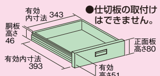
キャビネット1段付(NKL-S10□) キャビネット2段付(NKL-S20□) キャビネット3段付(NKL-S30□)
