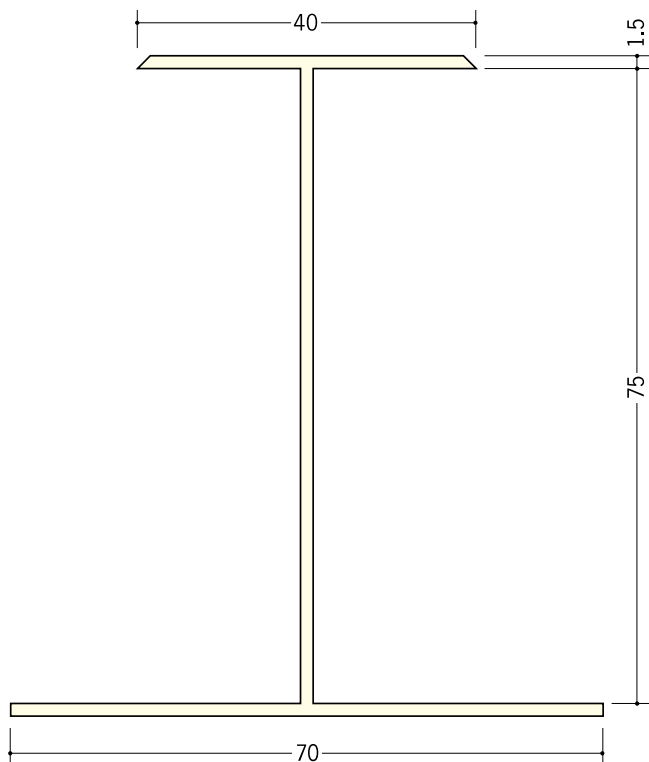
35093 H型75 2.73m/ホワイト・クリーム/各15本入
