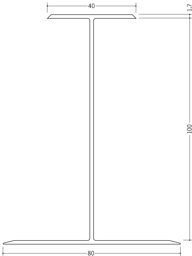
35094 H型100 2.73m/ホワイト・クリーム/各10本入
