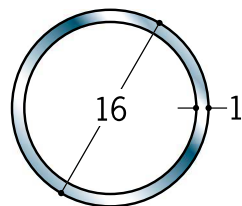
20115 ステン丸パイプ 16×1 2m/ヘアーライン
