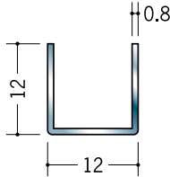
63143 ステンチャンネル 0.8×12×12 3m/ヘアライン
