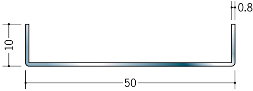
20122 ステンチャンネル 0.8×10×50 3m/ヘアライン
