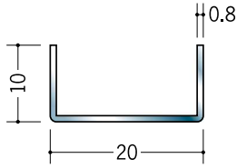
20021 ステンチャンネル 0.8×10×20 3m/ヘアライン
