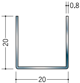
20023 ステンチャンネル 0.8×20×20 3m/ヘアライン
