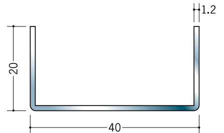
20027 ステンチャンネル 1.2×20×40 3m/ヘアライン
