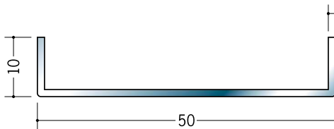
20124 ステンチャンネル 1.2×10×50 3m/ヘアライン
