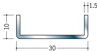
20026 ステンチャンネル 1.5×10×30 3m/ヘアライン
