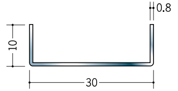
20022 ステンチャンネル 0.8×10×30 3m/ヘアライン
