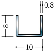
20019 ステンチャンネル 0.8×8×10 2m/ヘアライン
