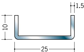
20025 ステンチャンネル 1.5×10×25 3m/ヘアライン
