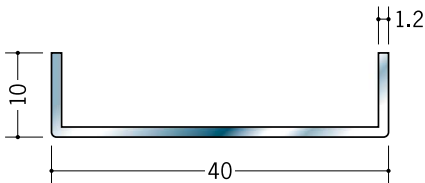
20123 ステンチャンネル 1.2×10×40 3m/ヘアライン
