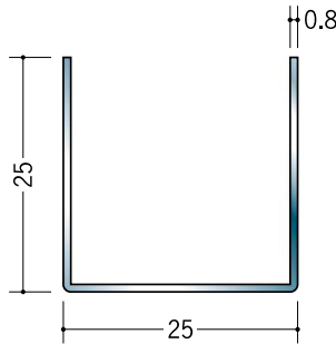
20020 ステンチャンネル 0.8×25×25 3m/ヘアライン
