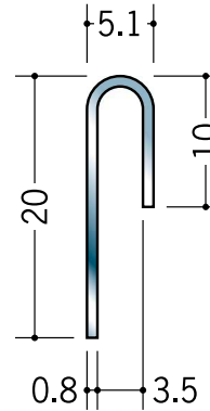
20113 ステンSUC-3.5 2m/へア-ライン t=0.8mm
