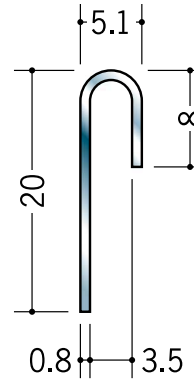
20108 ステンSUB-3.5 2m/へア-ライン t=0.8mm
