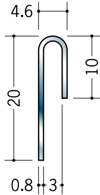
20112 ステンSUC-3 2m/へア-ライン t=0.8mm
