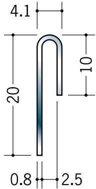
20111 ステンSUC-2.5 2m/へア-ライン t=0.8mm
