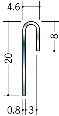
20107 ステンSUB-3 2m/へア-ライン t=0.8mm
