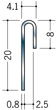
20106 ステンSUB-2.5 2m/へア-ライン t=0.8mm
