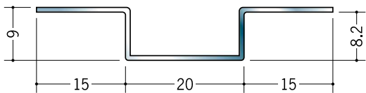
20087 ステンハット型 HE-20 2.73m/ヘアライン/t=0.8mm
