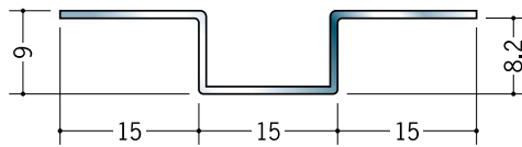
20086 ステンハット型 HE-15 2.73m/ヘアライン/t=0.8mm
