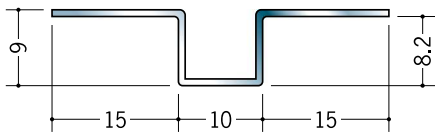
20085 ステンハット型 HE-10 2.73m/ヘアライン/t=0.8mm
