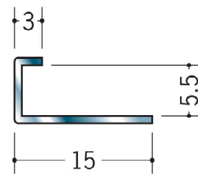
63283 ステン SCA-5 2m/ヘアーライン t=0.8mm
