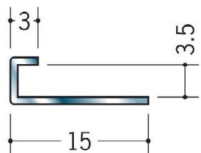
63281 ステン SCA-3 2m/ヘアーライン t=0.8mm
