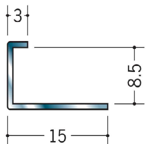
63285 ステン SCA-8 2m/ヘアーライン t=0.8mm
