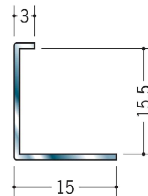
63288 ステン SCA-15 2m/ヘアーライン t=0.8mm
