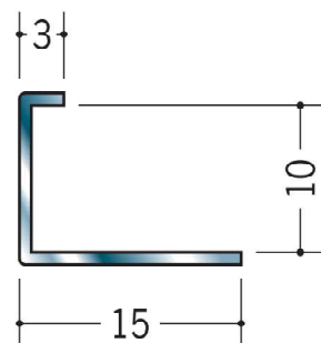
63286 ステン SCA-9 2m/ヘアーライン t=0.8mm
