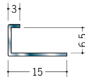
63284 ステン SCA-6 2m/ヘアーライン t=0.8mm
