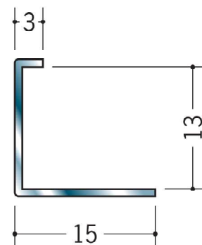
63287 ステン SCA-12 2m/ヘアーライン t=0.8mm
