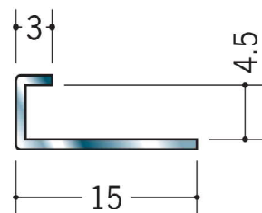
63282 ステン SCA-4 2m/ヘアーライン t=0.8mm
