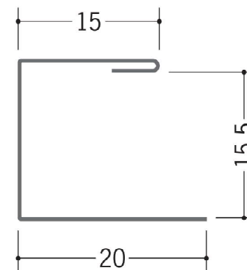
63206 コ型ハゼ付15.5 1.82m/アエンメッキ鋼板 t=0.27mm
