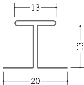
63215 H-13 1.82m/アインメッキ鋼板 t=0.27mm
