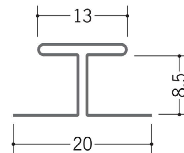
63213 H-8.5 1.82m/アインメッキ鋼板 t=0.27mm
