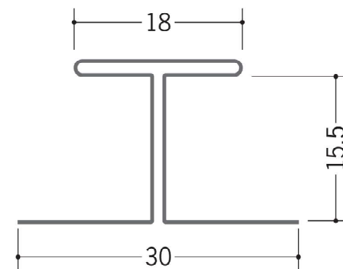
63216 H-15.5 1.82m/アインメッキ鋼板 t=0.27mm
