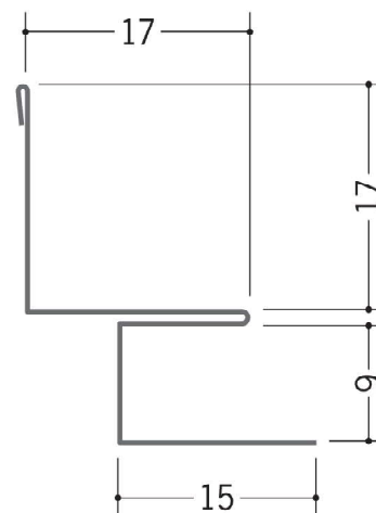
63158 亜鉛入隅8B 1.82m/アエンメッキ鋼板 t=0.27mm
