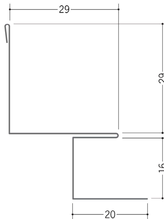
63161 亜鉛入隅15B 1.82m/アエンメッキ鋼板 t=0.27mm
