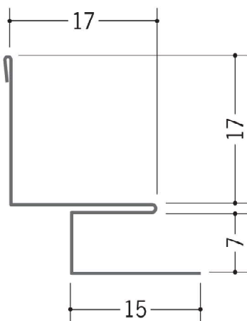
63157 亜鉛入隅6B 1.82m/アエンメッキ鋼板 t=0.27mm
