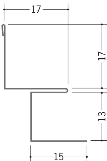
63160 亜鉛入隅12B 1.82m/アエンメッキ鋼板 t=0.27mm
