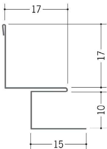
63159 亜鉛入隅9B 1.82m/アエンメッキ鋼板 t=0.27mm
