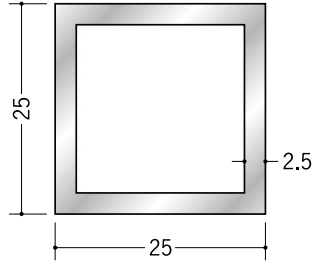
58066 アルミ角パイプ 2.5×25×25 2.5m (-3mm, +5mm) アルマイトシルバー
