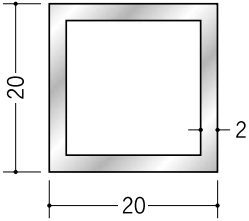
58064 アルミ角パイプ 2×20×20 2.5m (-3mm, +5mm) アルマイトシルバー
