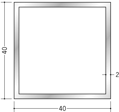
56319 アルミ角パイプ 2×40×40 2.5m (-3mm, +5mm) アルマイトシルバー
