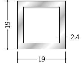
56315 アルミ角パイプ 2.4×19×19 2.4m / アルマイトシルバー
