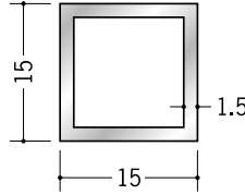
58063 アルミ角パイプ 1.5×15×15 2.5m (-3mm, +5mm) アルマイトシルバー
