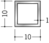
56313 アルミ角パイプ 1×10×10 2.5m (-3mm, +5mm) アルマイトシルバー
