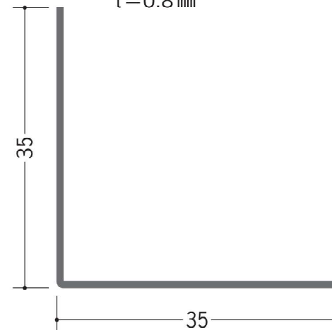
63196 ボンデアングル 0.8×35×35 1.82m/ボンデ鋼板 t=0.8 mm
