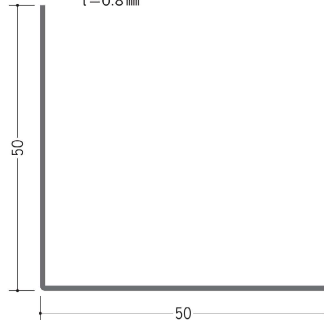
63199 ボンデアングル 0.8×50×50 1.82m/ボンデ鋼板 t=0.8 mm
