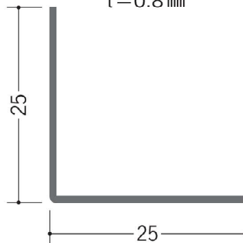
63194 ボンデアングル 0.8×25×25 1.82m/ボンデ鋼板 t=0.8 mm
