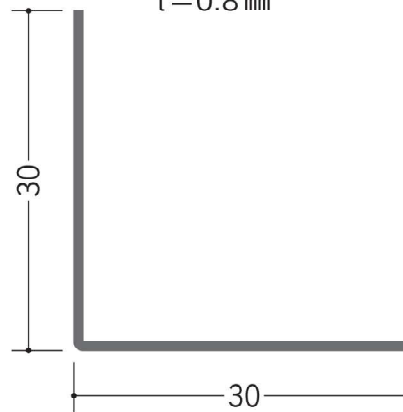
63195 ボンデアングル 0.8×30×30 1.82m/ボンデ鋼板 t=0.8 mm
