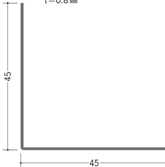
63198 ボンデアングル 0.8×45×45 1.82m/ボンデ鋼板 t=0.8 mm
