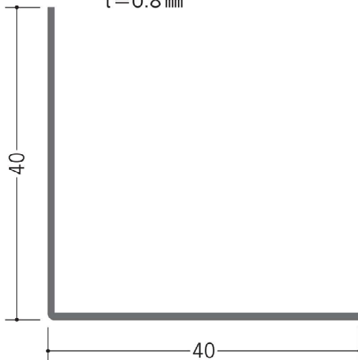
63197 ボンデアングル 0.8×40×40 1.82m/ボンデ鋼板 t=0.8 mm
