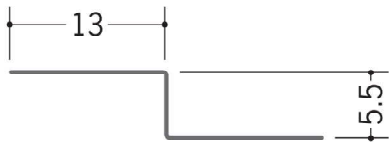
63241 水切 5 1.82m/アエンメッキ鋼板 t=0.27mm
