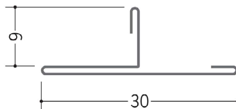
63255 TCK30-9 1.82m/アエンメッキ鋼板 t=0.27mm
