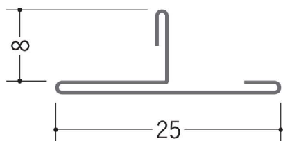
63251 TCK25-8 1.82m/アエンメッキ鋼板 t=0.27mm
