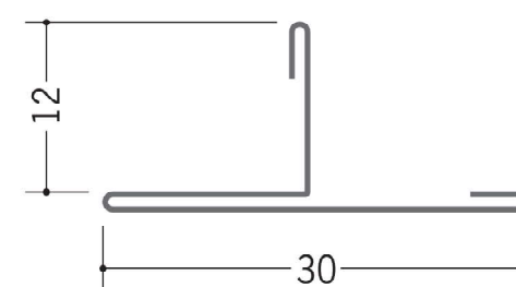
63252 TCK30-12 1.82m/アエンメッキ鋼板 t=0.27mm
