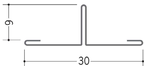
63253 TCW30-9 1.82m/アエンメッキ鋼板 t=0.27mm
