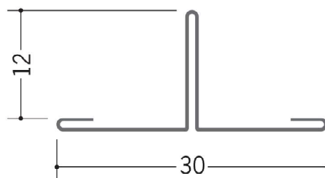
63254 TCW30-12 1.82m/アエンメッキ鋼板 t=0.27mm
