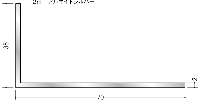
56276 アルミアングル 2×35×70 2m/アルマイトシルバー
