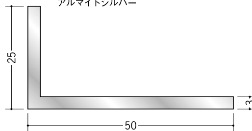
56165 アルミアングル 3×25×50 2m (-3mm, +5mm) アルマイトシルバー
