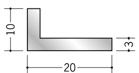
56174 アルミアングル 3×10×20 2m/アルマイトシルバー
