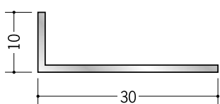
56144 アルミアングル 1.2×10×30 3m/アルマイトシルバー
