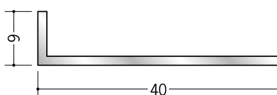
56136 アルミアングル 1.5×9×40 3m/アルマイトシルバー
