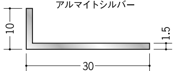
56262 アルミアングル 1.5×10×30 2m(-3mm, +5mm) アルマイトシルバー
