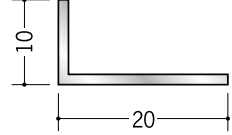
56142 アルミアングル 1.2×10×20 3m/アルマイトシルバー
