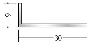
56134 アルミアングル 1.2×9×30 3m/アルマイトシルバー
