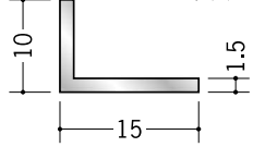
56132 アルミアングル 1.5×10×15 2m(-3mm, +5mm) アルマイトシルバー
