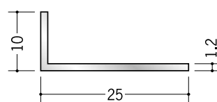
56072 アルミアングル 1.2×10×25 3m/アルマイトシルバー
