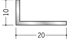
56260 アルミアングル 1.5×10×20 2m(-3mm, +5mm) アルマイトシルバー
