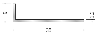
56135 アルミアングル 1.2×9×35 3m/アルマイトシルバー
