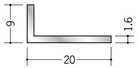
56076 アルミアングル 1.6×9×20 3m/アルマイトシルバー
