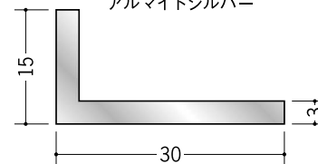
56177 アルミアングル 3×15×30 2m (−3mm, +5mm) アルマイトシルバー
