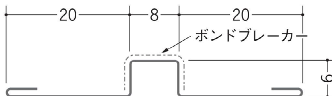
63272 サイディングジョイナー 6×8 1.82m / アエンメッキ鋼板 / t=0.27mm
