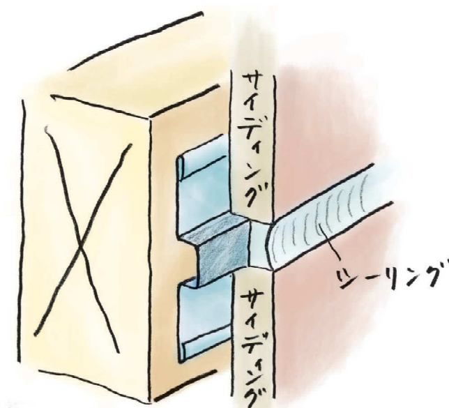
63272 サイディングジョイナー 6×8 1.82m / アエンメッキ鋼板 / t=0.27mm
