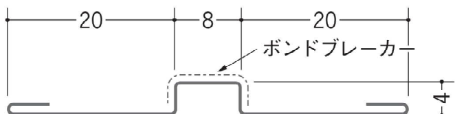
63271 サイディングジョイナー 4×8 1.82m / アエンメッキ鋼板 / t=0.27mm
