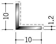
29093 アルミカラーアングル 1.2×10×10入隅用 3m／パニラホワイト カスタムブラック
