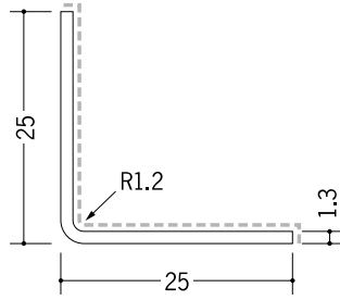
29092 アルミカラーアングル L2R25×25入隅用 3m／パニラホワイト カスタムブラック
