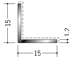
29095 アルミカラーアングル 1.2×15×15入隅用 3m／パニラホワイト カスタムブラック
