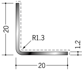
29091 アルミカラーアングル L2R20×20入隅用 3m／パニラホワイト カスタムブラック
