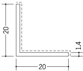
29096 アルミカラーアングル 1.4×20×20入隅用 3m／パニラホワイト カスタムブラック
