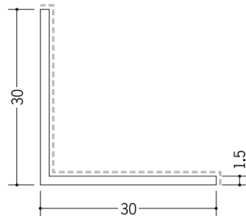
29098 アルミカラーアングル 1.5×30×30入隅用 3m／パニラホワイト カスタムブラック
