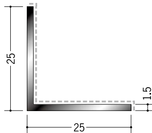
29097 アルミカラーアングル 1.5×25×25入隅用 3m／パニラホワイト カスタムブラック
