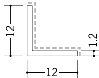
29094 アルミカラーアングル 1.2×12×12入隅用 3m／パニラホワイト カスタムブラック
