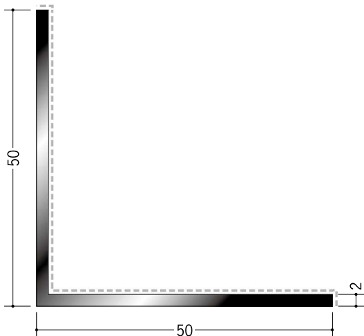
29099 アルミカラーアングル 2×50×50入隅用 3m／パニラホワイト カスタムブラック
