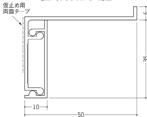
34501 シーリングアングルPCL-50 2m/オフホワイト/t=1.5mm
