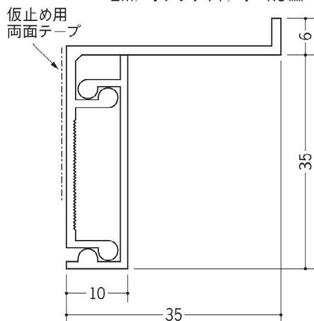
34500 シーリングアングルPCL-35 2m/オフホワイト/t=1.5mm
