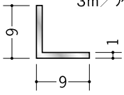
56021 アルミアングル 1×9×9 3m/アルマイトシルバー
