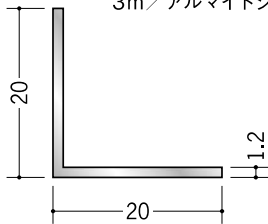
アルミアングル 1.2×20×20 3m/アルマイトシルバー
