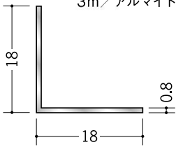
56036 アルミアングル 0.8×18×18 3m/アルマイトシルバー
