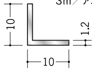
56022 アルミアングル 1.2×10×10 3m/アルマイトシルバー
