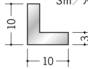
アルミアングル 3×10×10 3m/アルマイトシルバー
