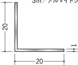
56106 アルミアングル 1×20×20 3m/アルマイトシルバー
