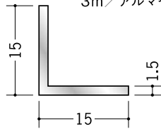
アルミアングル 1.5×15×15 3m/アルマイトシルバー
