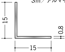
56034 アルミアングル 0.8×15×15 3m/アルマイトシルバー
