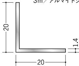
アルミアングル 1.4×20×20 3m/アルマイトシルバー
