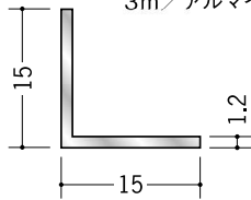
アルミアングル 1.2×15×15 3m/アルマイトシルバー
