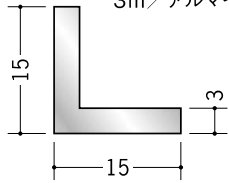
アルミアングル 3×15×15 3m/アルマイトシルバー
