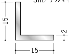
56114 アルミアングル 2×15×15 3m/アルマイトシルバー
