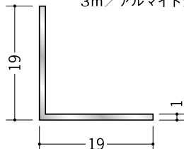
56024 アルミアングル 1×19×19 3m/アルマイトシルバー
