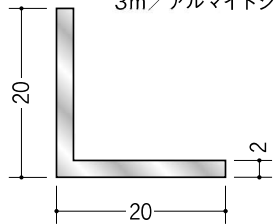
アルミアングル 2×20×20 3m/アルマイトシルバー
