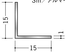
アルミアングル 1×15×15 3m/アルマイトシルバー
